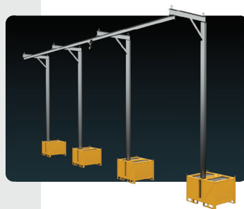
10 Conjunto de Postes Linha de Vida Com caixa contrapeso
